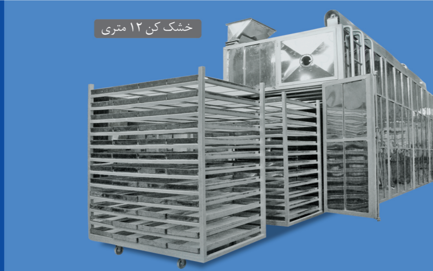
مجموعه خشک کن با منبع حرارتی بایومس
